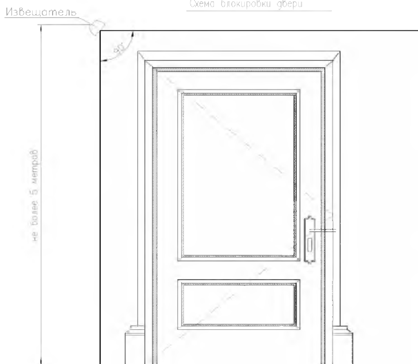
Схема блокировки двери
